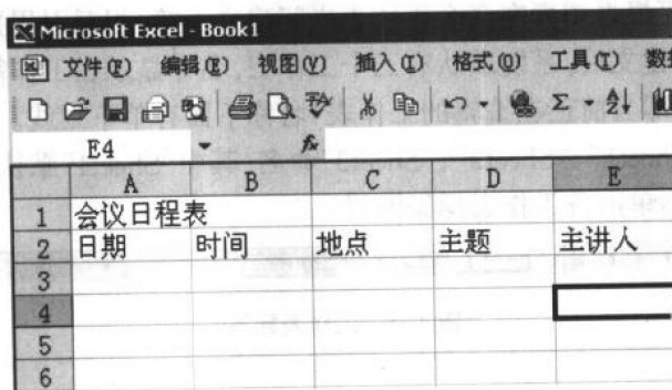
图 1.9 输入列标题
