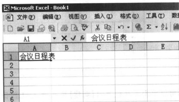
图 1.8 输入标题
