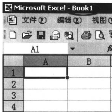
图 1.6 新建工作簿
