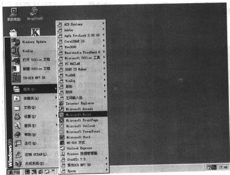
图 1.2 启动 Excel 2002
