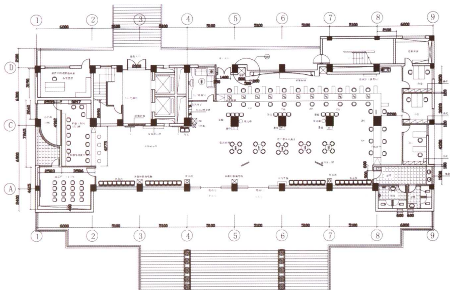
一层平面图
