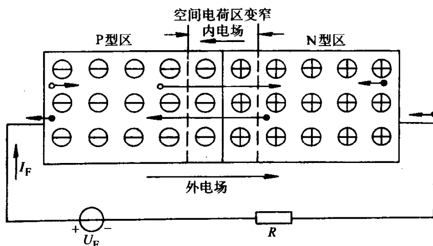
图 1-6 外加正向电压的 PN 结
