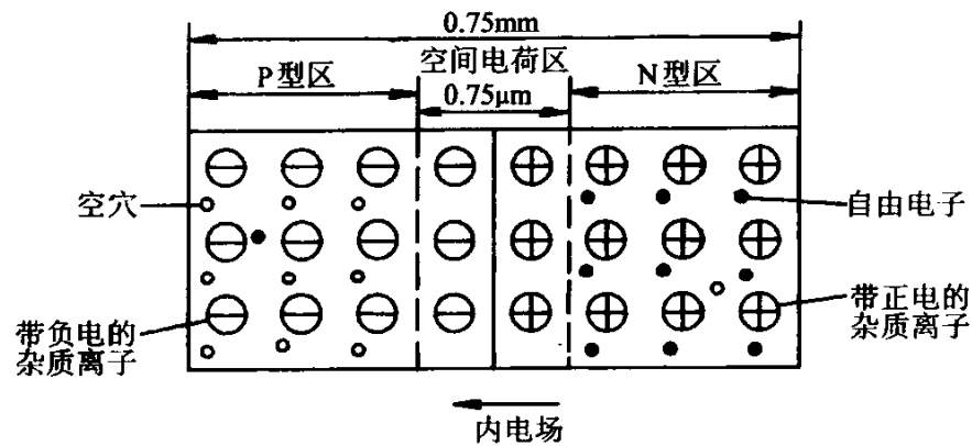
图 1-5 PN 结的形成
