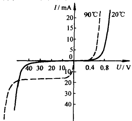
图 1-11 温度对二极管伏安特性的影响
