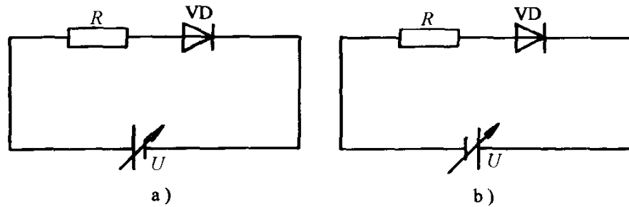
图1-9 二极管伏安特性测试电路
