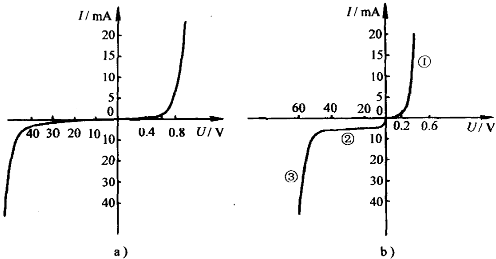
图1-10 二极管的伏安特性曲线
