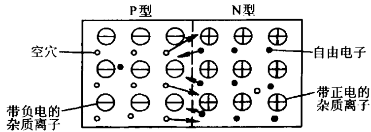
图 1-4 载流子的扩散
