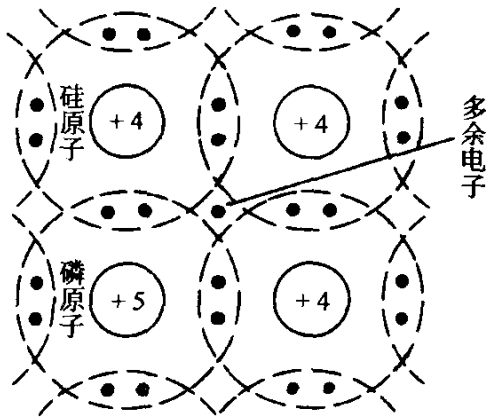
图 1-2 N 型半导体的共价键结构
