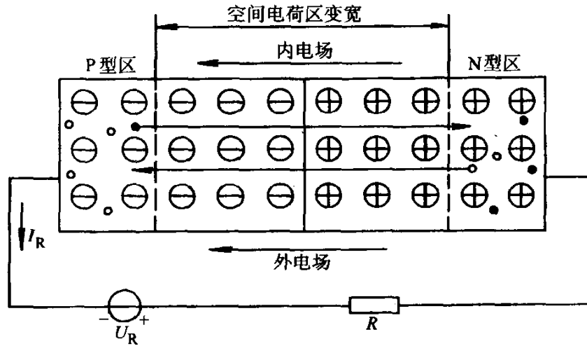
图 1-7 外加反向电压的 PN 结
