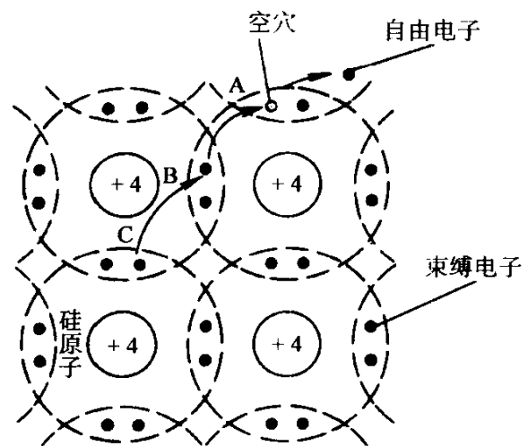
图 1-1 电子和空穴的移动
