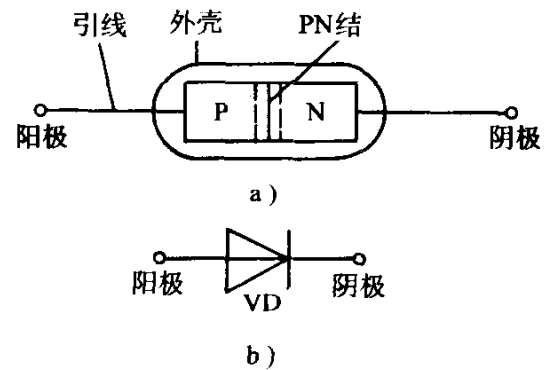
图1-8 二极管的结构示意图和图形符号
