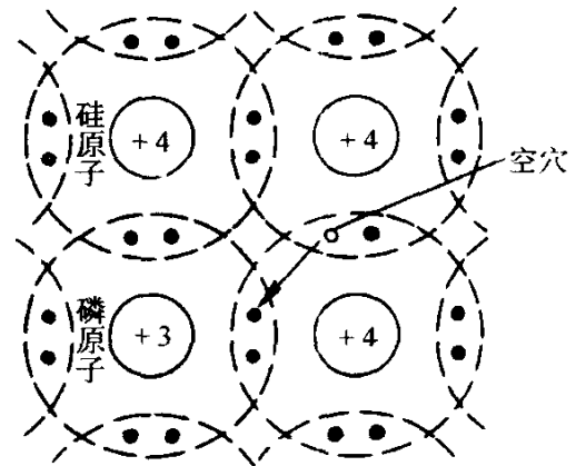
图 1-3 P 型半导体的共价键结构
