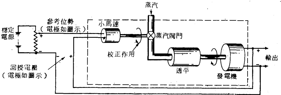
圖 1.3 具有自動誤差校正之簡單調節器圖。
