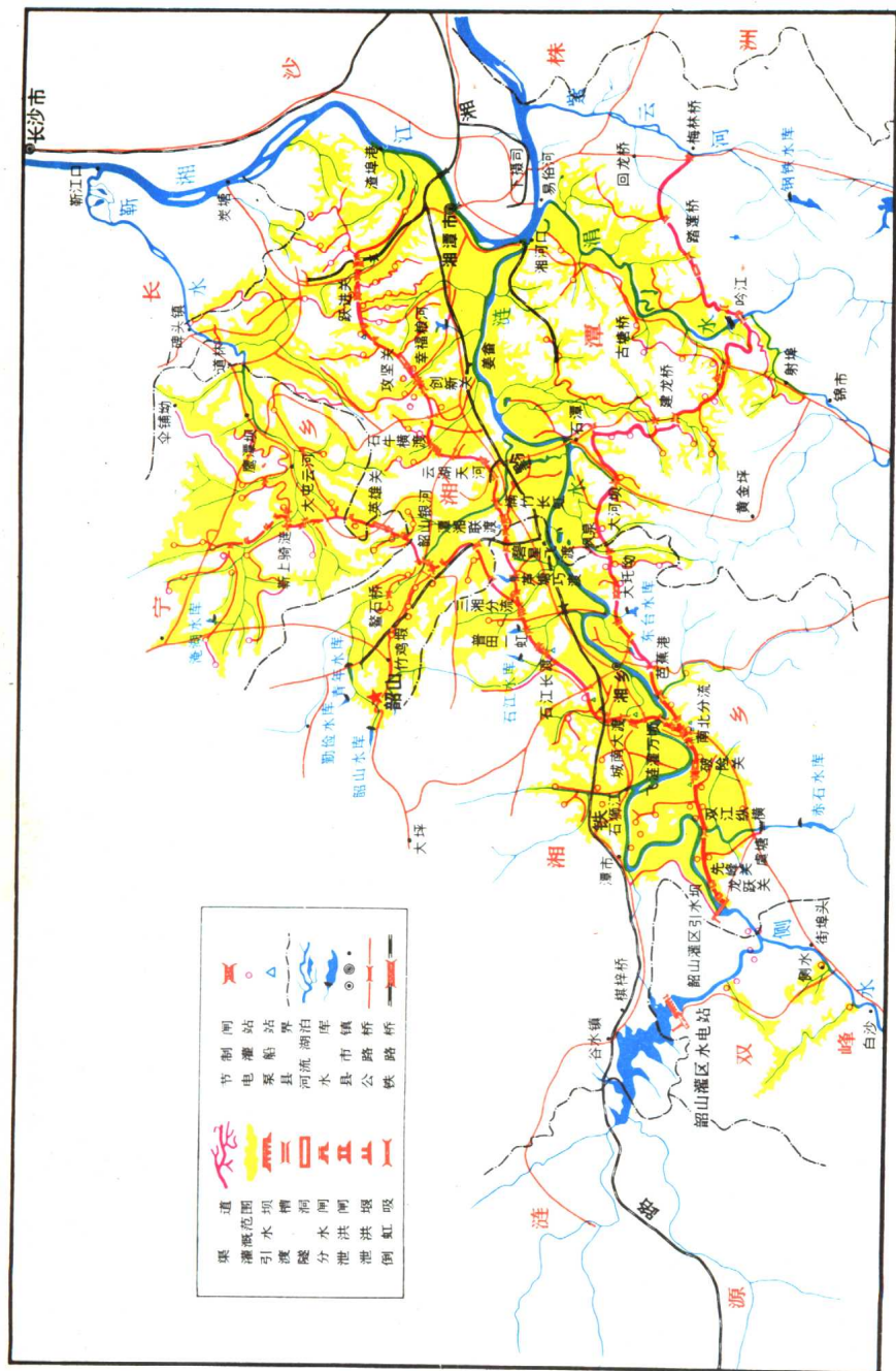
韶山灌区示意图
