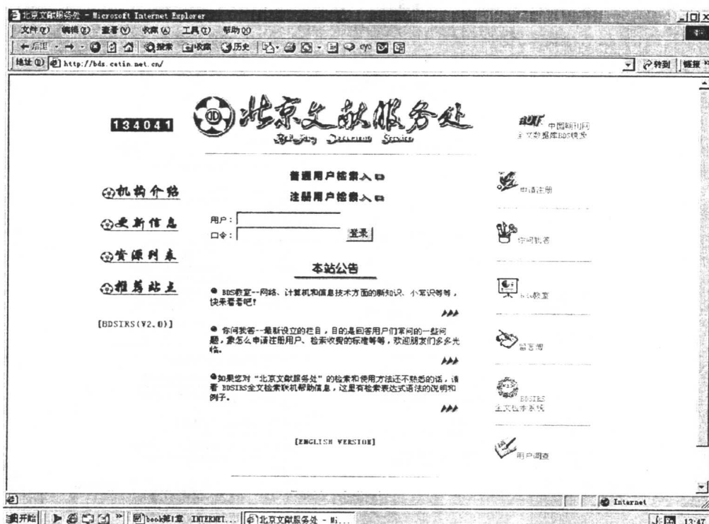
图 1.8 BDS 主页
