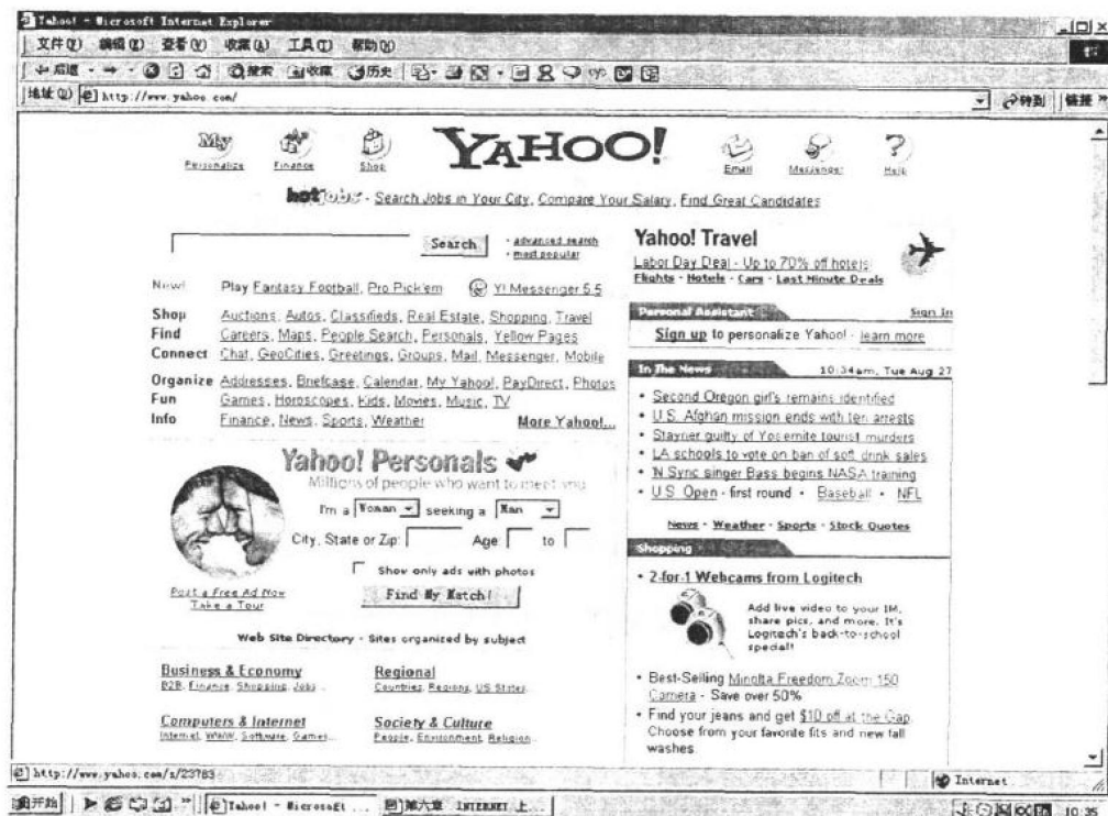
图 1.9 Yahoo 主页
