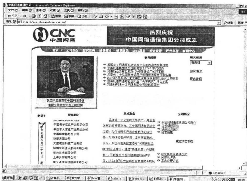
图 1.5 ChinaNET 主页
