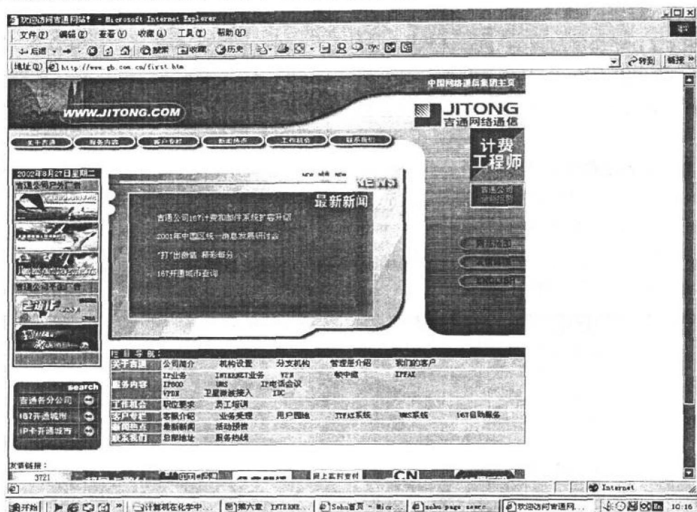
图 1.6 金桥网主页
