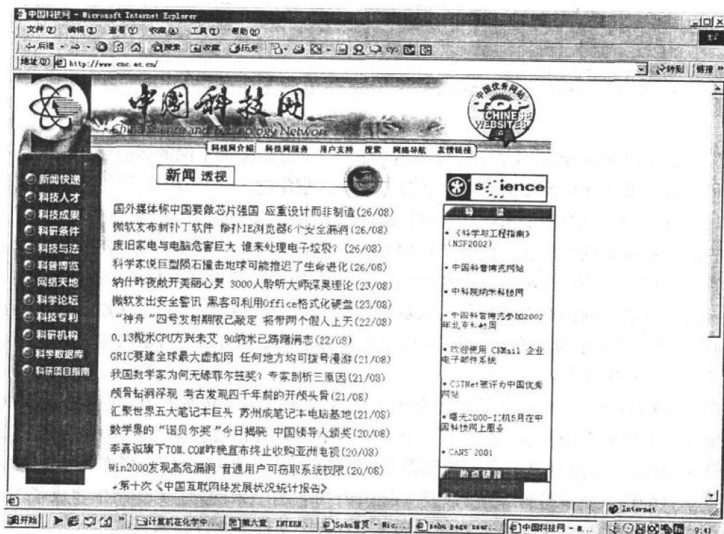
图 1.3 CASNET 主页
