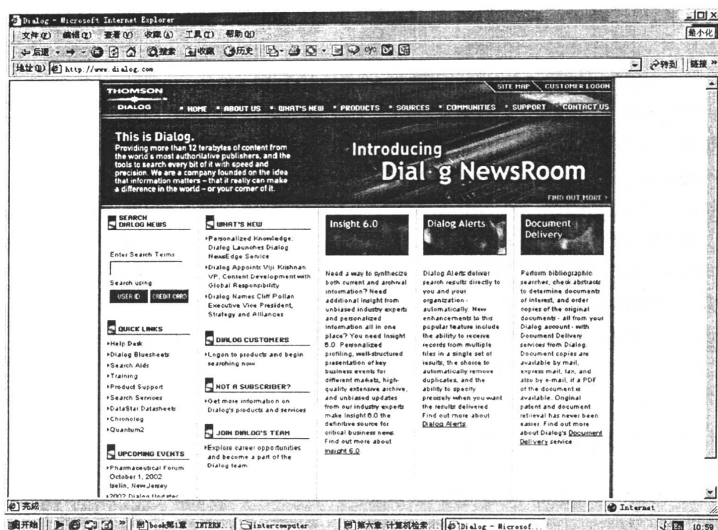
图 1.7 DIALOG 主页
