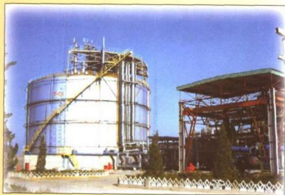
扬子石化公司从德国引进的10000m 3 低温乙烯储存装置 (1998年荣获国家建筑工程鲁班奖) 项目经理:刘天应
