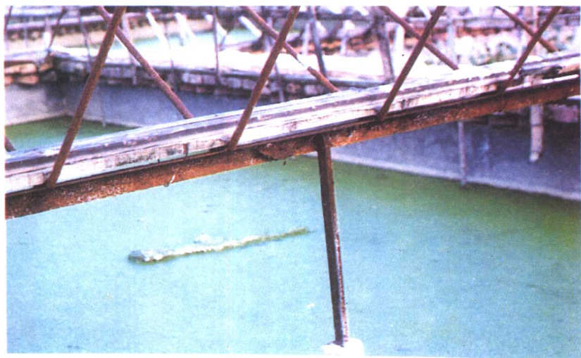
图 13 悬空棚脚及立柱
