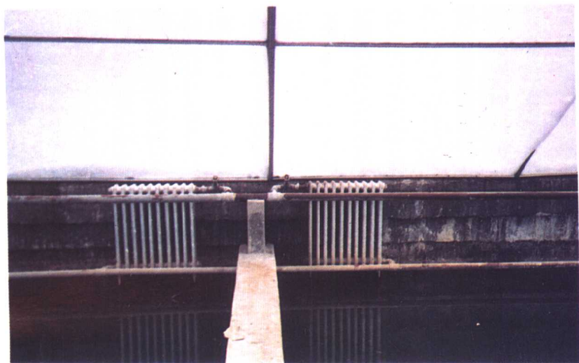
图 17 温室内散热器
