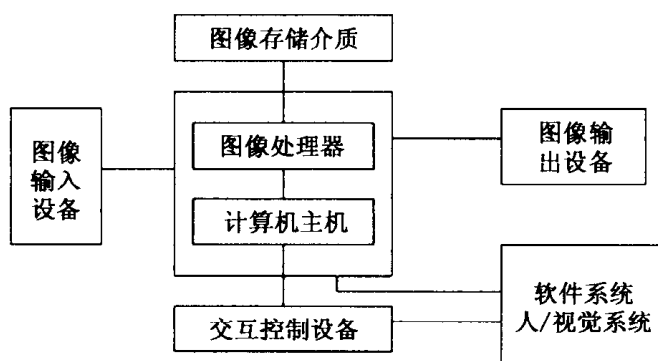
图 1-1 典型数字图像处理系统框图
