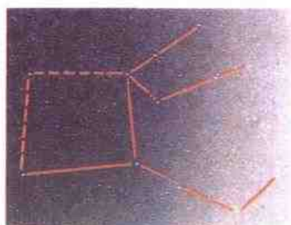
飞马座
