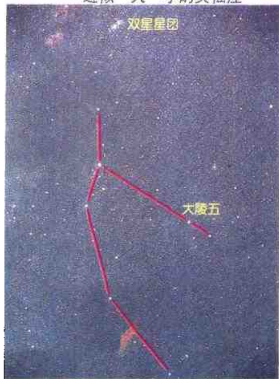
英仙座
