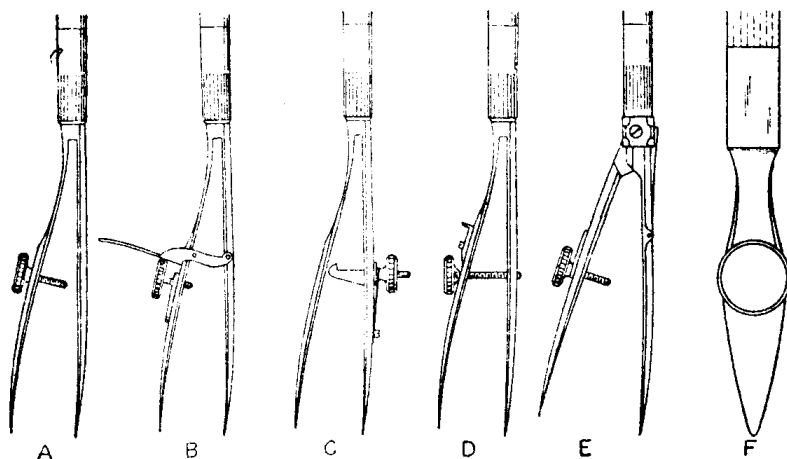
圖 2.7 直線筆。開口以便去污。
