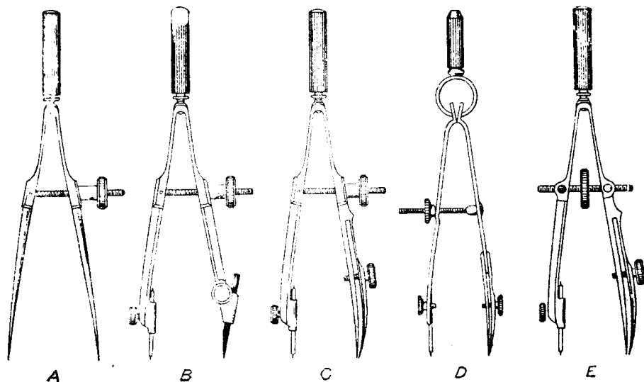
圖 2.6 彈簧弓形儀器 (Spring Bow Instruments)。
