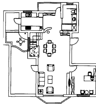
二楼现状平面图
