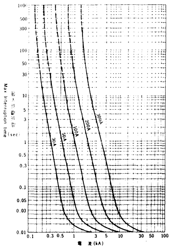
圖 1-5 : OF 型最大啓斷時間—電流特性 ( OF Type Max. Interruption time-Current characteristics )
