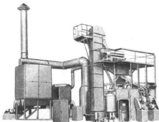
Q7710型抛喷丸落砂清理室
