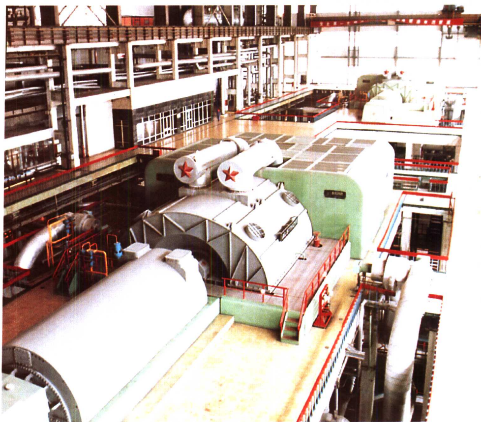
1985、1986 年投产的 3、4 号 30 万千瓦汽轮发电机组
