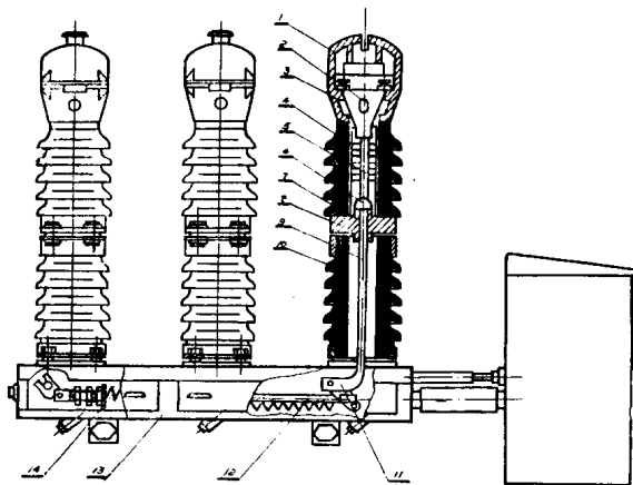
SW2—35少油断路器结构示意图
