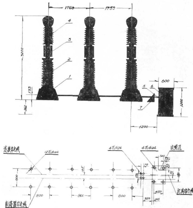
图二 断路器单极外形图(110KV)
