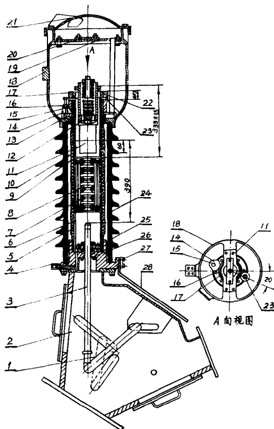
图一 断路器断口剖面图
