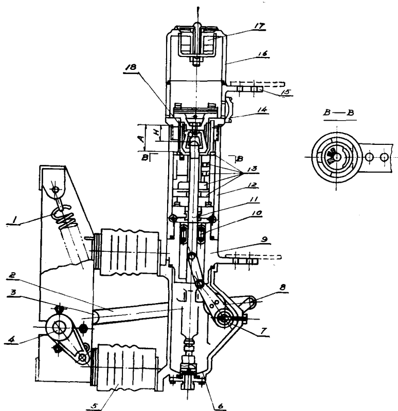
SN10少油断路器结构示意图
