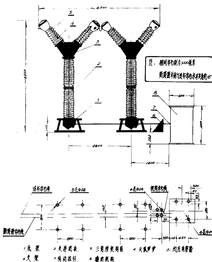
图四 外形及安装尺寸(220KV)
