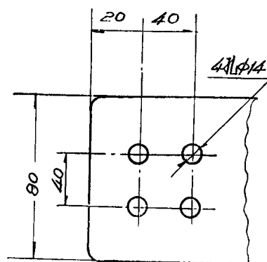
SN10—10/1000-500 接线端尺寸图
