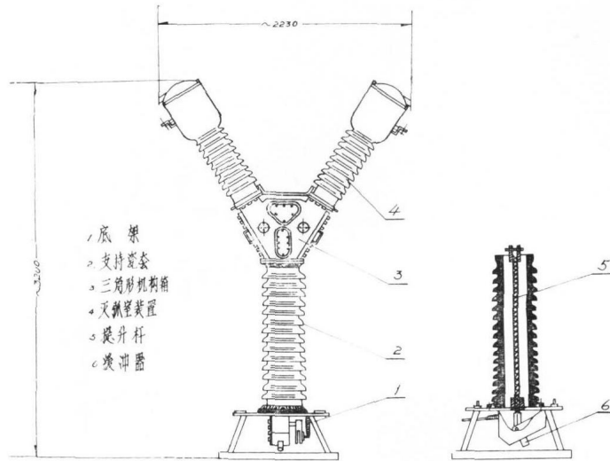
图二 断路器单极外形图(110KV)
