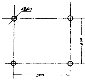
断路器安装尺寸图
