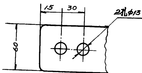
SN10—10/600-300接线端尺寸图
