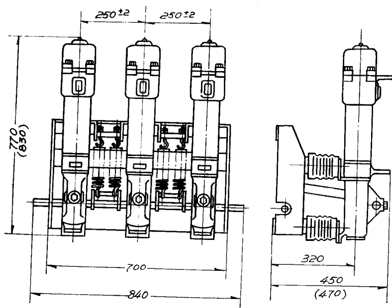
SN10—10 断路器外形图
