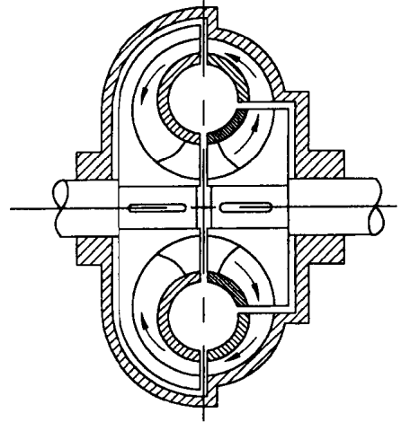
图 0-8 液力变矩器
