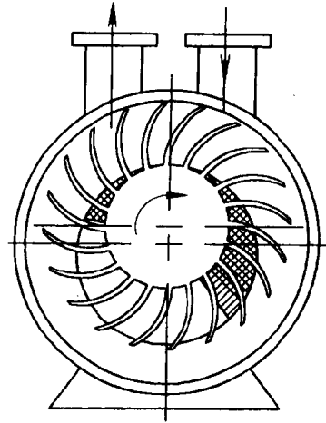
图 0-4 液环式流体机械
