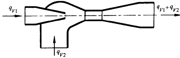
图 0-3 射流泵
