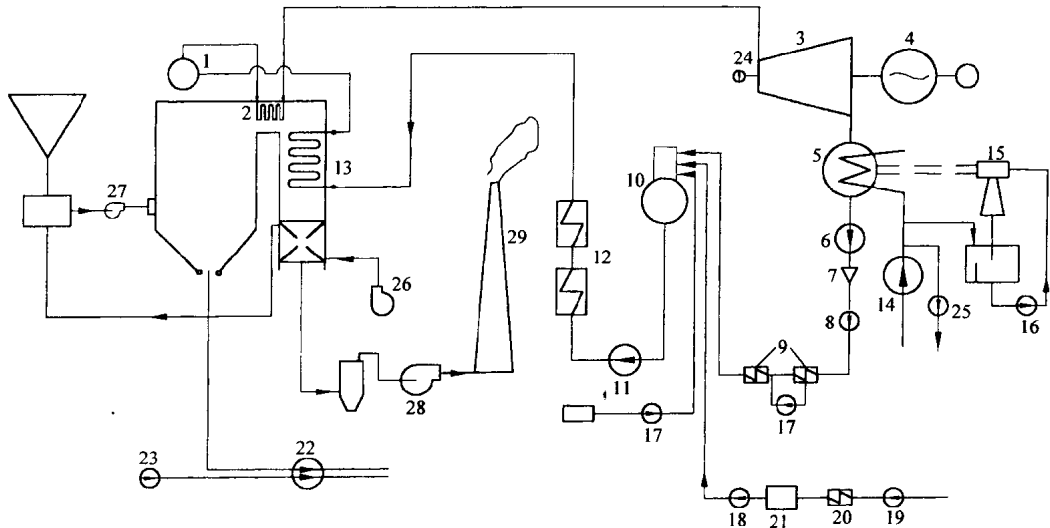
图 0-5 热力发电厂系统简图
