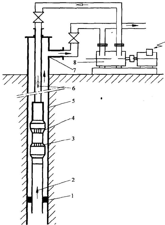
图 0-7 水下油气混输泵装置
