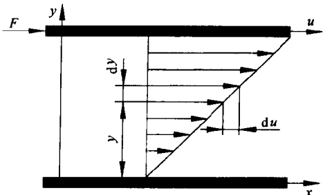
图 0-10 流体的粘度
