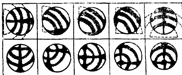
圖 2. 一軸晶近于垂直光軸的斜切面內的錐光圖
