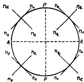
圖 3. 在一軸晶垂直于光軸的切面內, 常光及非常光的振動方向
