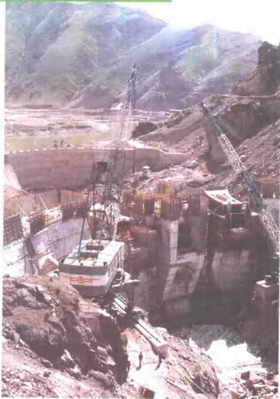
建设中的巴音郭楞蒙古自治州大山口水电站(装机 4\times 2 万千瓦)
