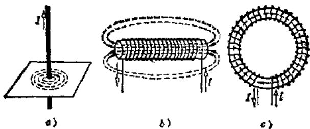
图1-11 通电导线周围的磁场
