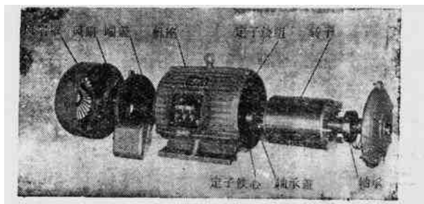
图1-2 三相异步电动机的构造
