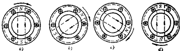
图1-13 三相交流电产生的旋转磁场
