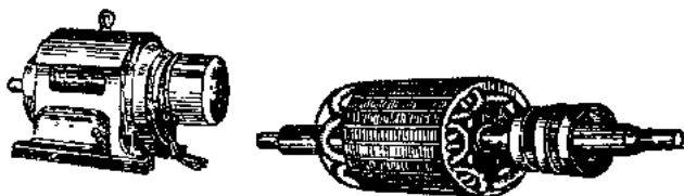
图1-6 绕线式电动机外形和绕线转子
