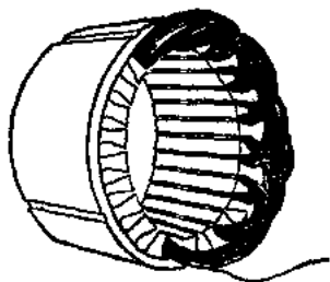
图1-3 定子铁心和定子绕组
