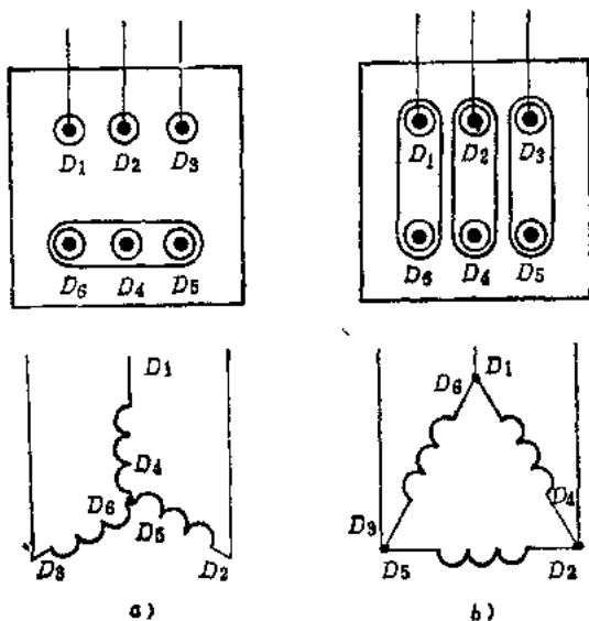
图 1-4 三相绕组的连接
