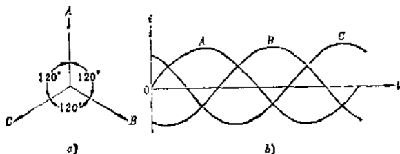
图1-12 三相交流电
