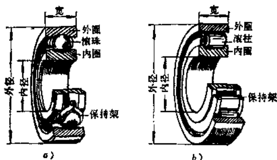
图1-10 滚动轴承的构造
