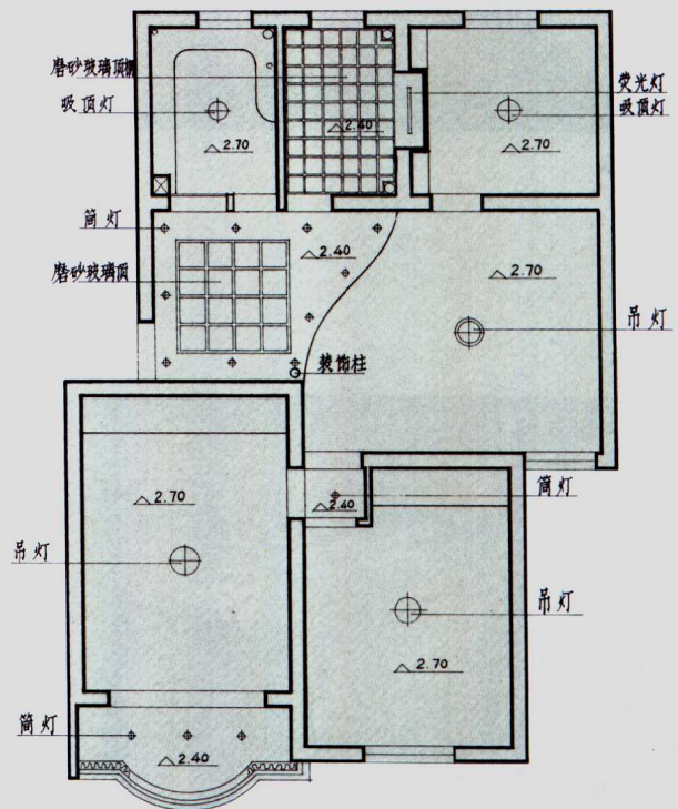
平顶图
