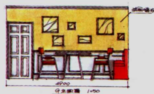
F 立面图 1250
