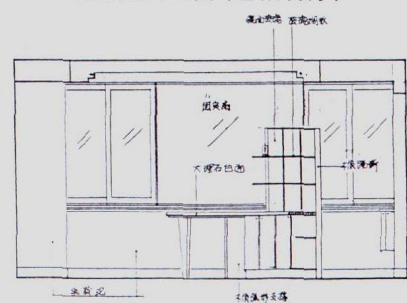
客、餐厅D立面
