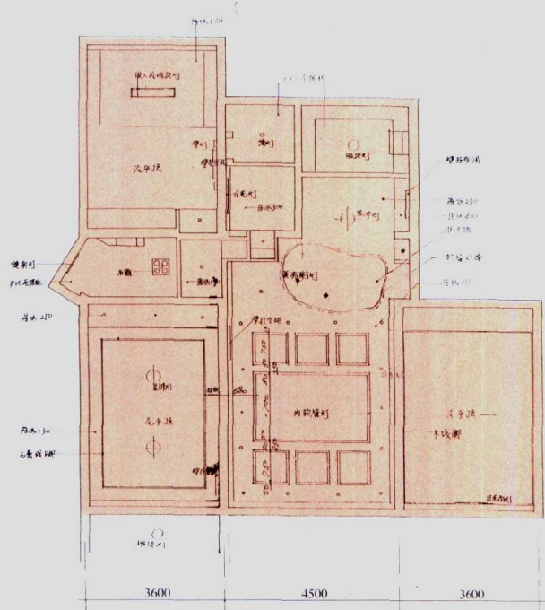
平面图
