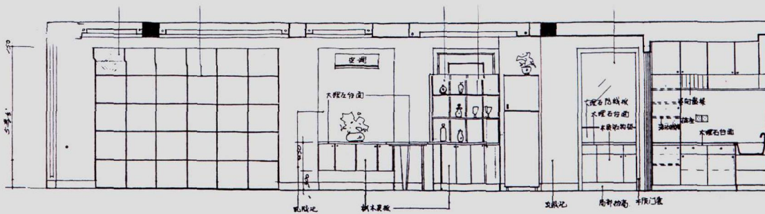
客、餐厅A立面 (包括厨房)
