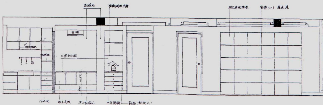
客、餐厅C立面
