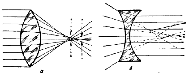
圖4 球面像差
