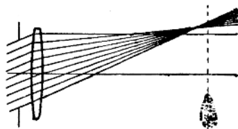
圖6 偏向光綫的像差（彗形像差）
