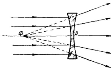
圖3 在發散透鏡中的光程
