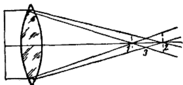
圖 10 色差
