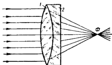
圖5 消球面像差系統
