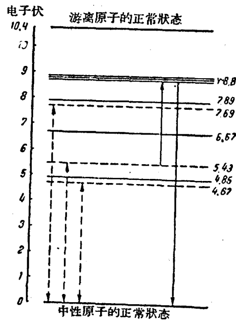
圖 1-2 汞原子的低級能級 虛綫表示介穩能級，虛箭头表示被禁止的轉变，实箭头表示某些可容許的轉变。
