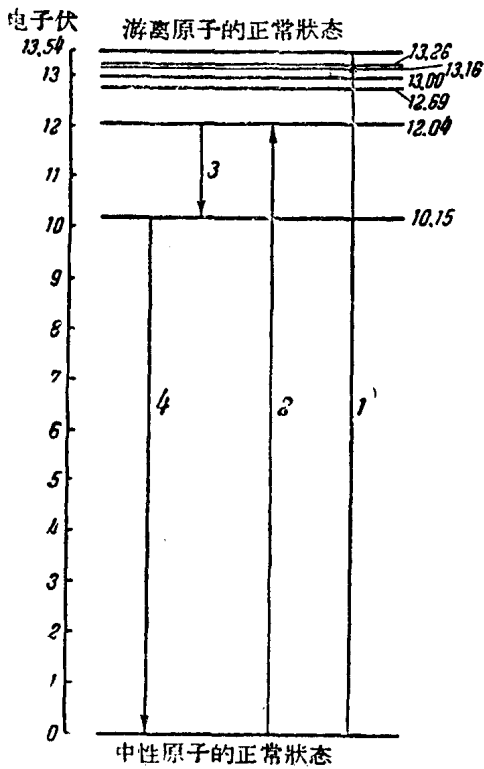
圖 1-1 氫原子的能級 各箭头指示：1—耗能 13.54 电子伏而游离；2—耗能 12.04 电子伏而激發；3—由高軌道轉到低軌道，放出能 1.9 电子伏(波長 656.3 毫微米)；4—激發原子恢复正常状态，放出能 10.15 电子伏(波長 121.6 毫微米)。
