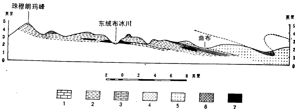
图1 珠穆朗玛峰北坡地质剖面图(Wager, 1934)
