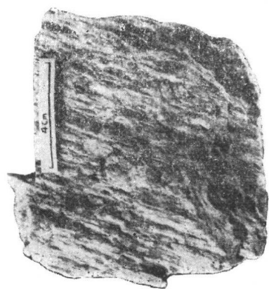
1. 受强烈破碎的白云母花岗岩片麻岩(花岗岩质压碎岩)(标本号 Js-11)
