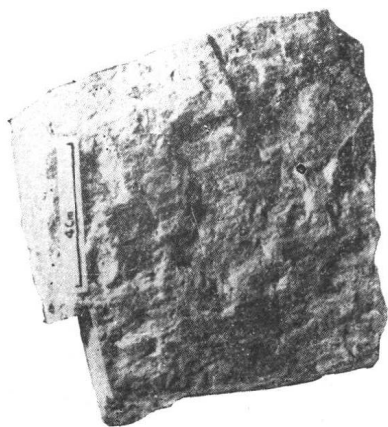
2. 受强烈破碎的白云母花岗岩片麻岩(花岗岩质压碎岩)(标本号 Jk-15)
