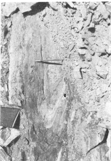
7. 黄带层条状大理岩中的倒转褶皱(秋哈拉沟, 镜头向西照)
