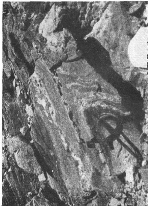
4. 绒布组顶部黑石英片岩中的向南倒转的褶皱(基龙贡巴南山, 镜头向东照)
