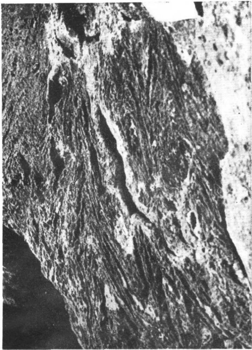
5. 绒布组顶部大理岩中的向南倒转及平卧的褶皱(基龙贡巴南山, 镜头向东照)
