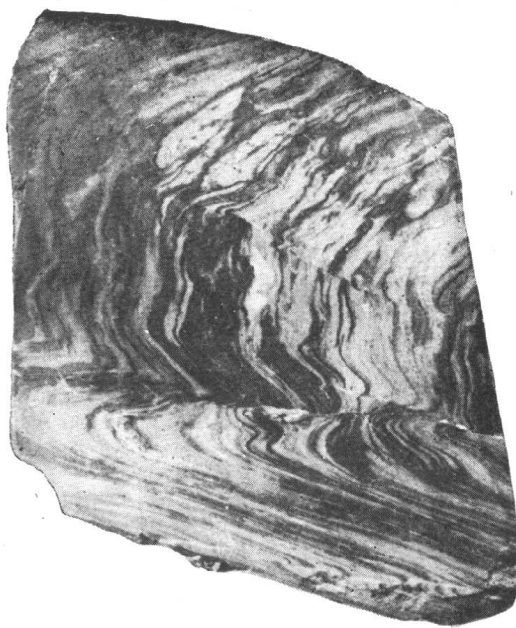
10. 黄带层条状大理岩中的褶皱和小型逆掩断层(转石)(秋哈拉沟)
