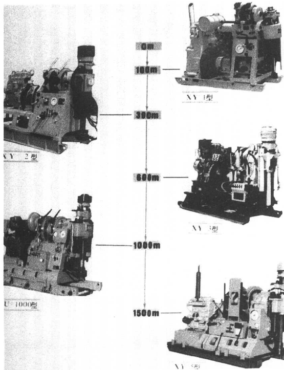
地矿部门岩心钻机系列
