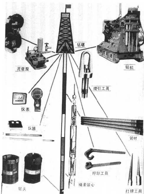
金刚石钻探配套技术装备
