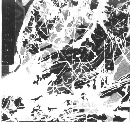
地质矿产图与航磁等值线、遥感 线性体、环性体叠合显示图
