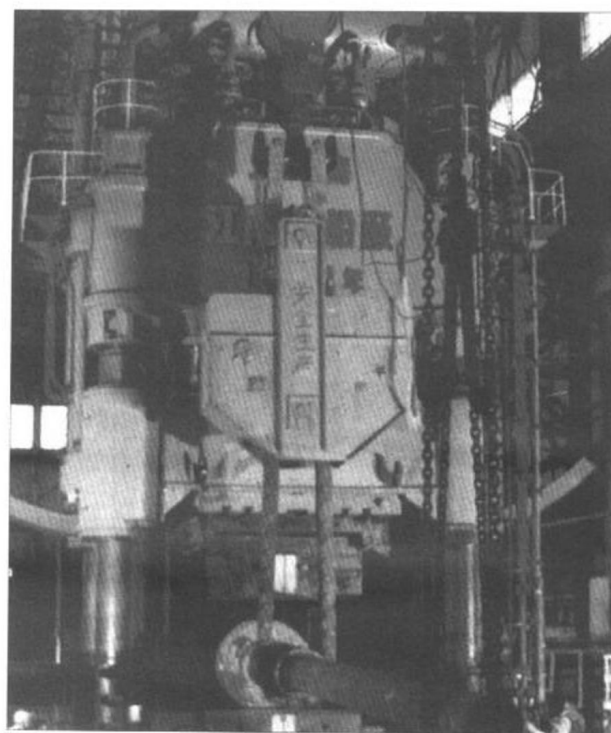
1961年，上海江南造船厂制造成功1.2万吨水压机，标志着中国重型机器制造业达到了新的水平(上图)。
