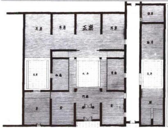
圖 1-8 大夫第平面圖
