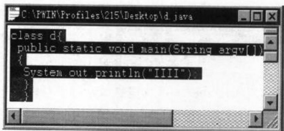
图 3-1 选取块
