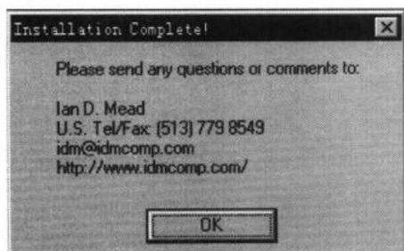
图 1-4 安装完成
