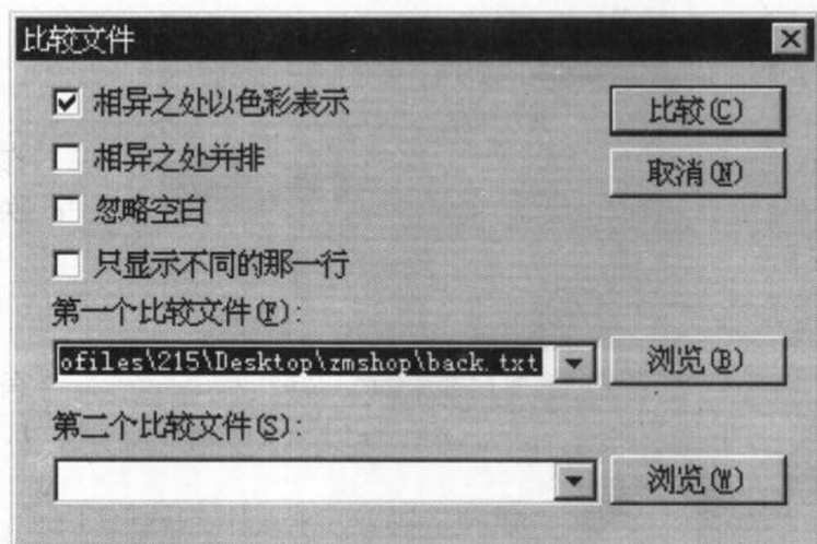
图 2-2 比较文件
