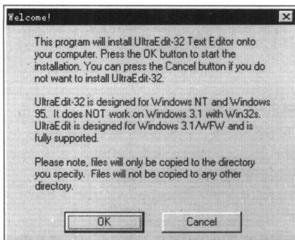
图 1-1 欢迎对话框
