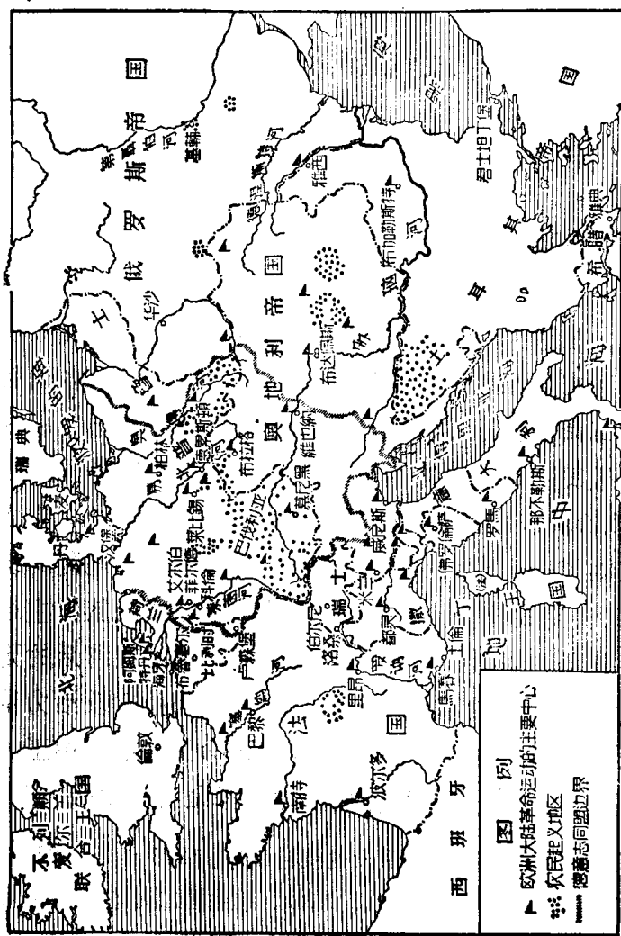
1848年欧洲革命
