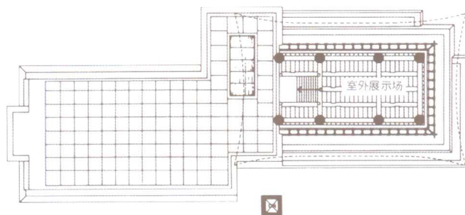
屋顶层平面图
