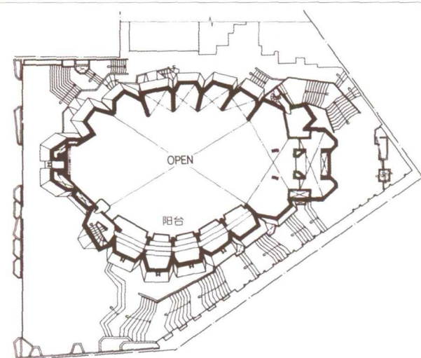
上层平面图
