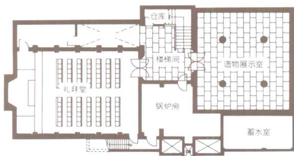
地下层平面图
