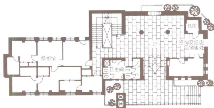
1层平面图
