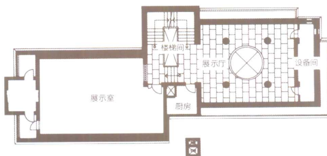
2层平面图
