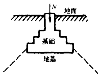
图 1-1 地基及基础示意图
