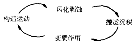
图 2-1 地质循环示意图
