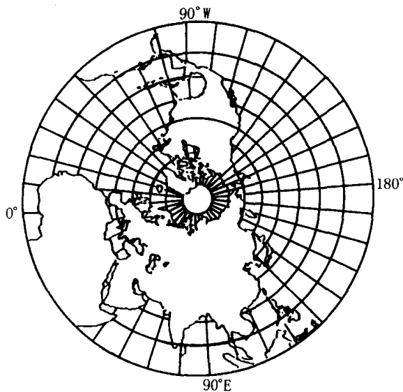
图 1.4 极射赤道投影北半球图
