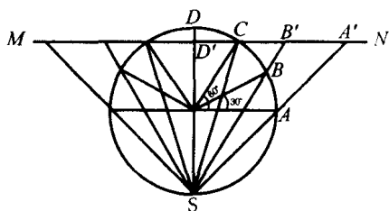
图 1.3 极射赤道投影法
