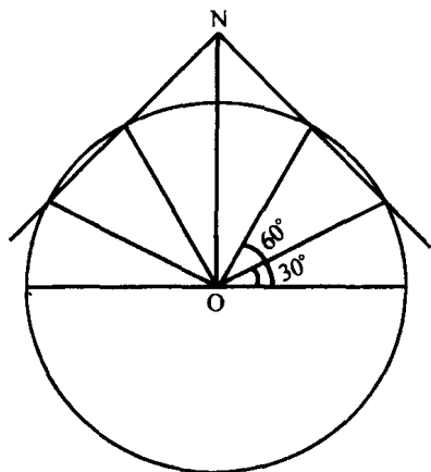
图 1.1 双标准纬圈圆锥投影法
