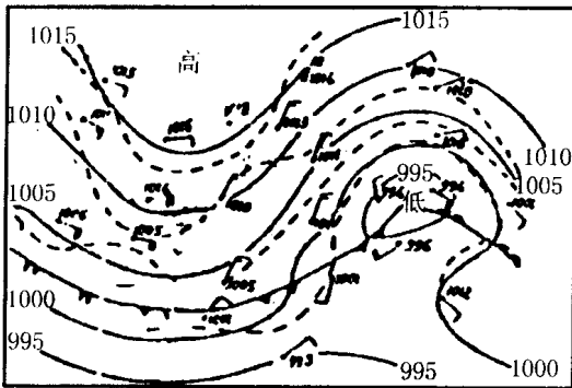
图 1.12 等压线画法
