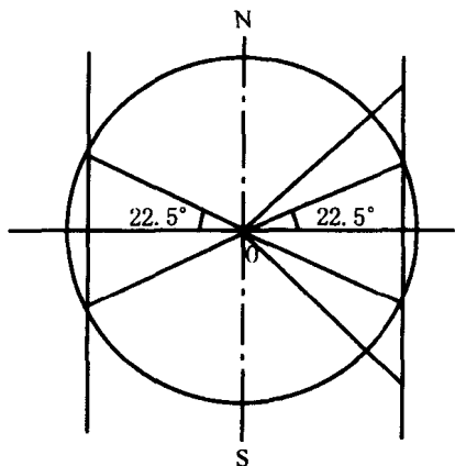
图 1.5 墨卡托投影法
