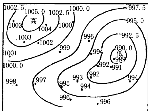
图 1.8 海平面等压线图
