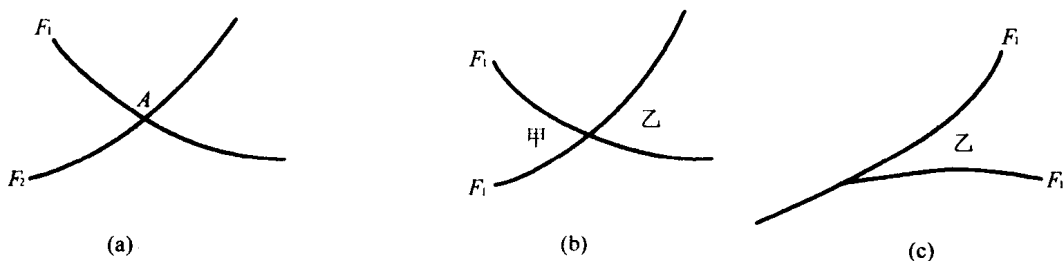
图 1.9 等压线的错误分析
