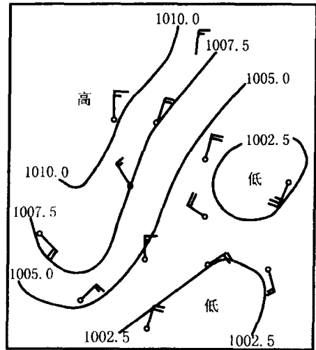
图 1.11 等压线与风的关系
