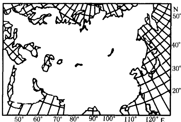
图 1.2 兰勃特投影图
