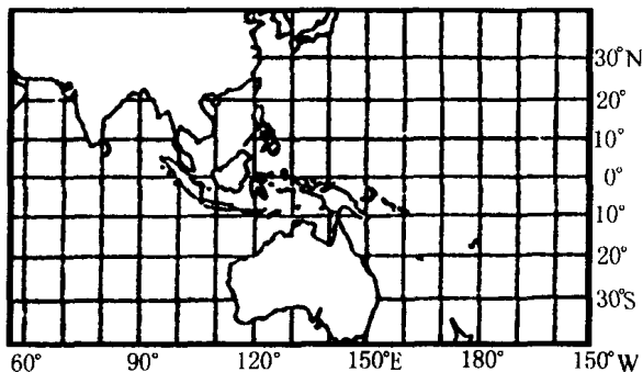
图 1.6 墨卡托投影图
