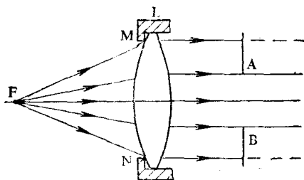
图7-2 孔径光栏在透镜之后
