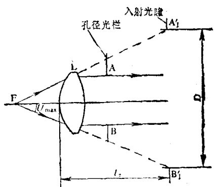
图7-3 入射光瞳和物方孔径角的示意图
