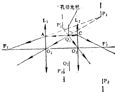
图7-5 用作图法求光学系统的入瞳和出瞳
