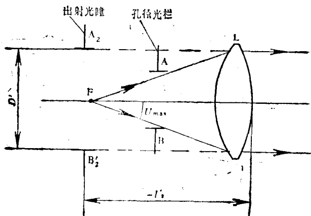
图7-4 出射光瞳示意图
