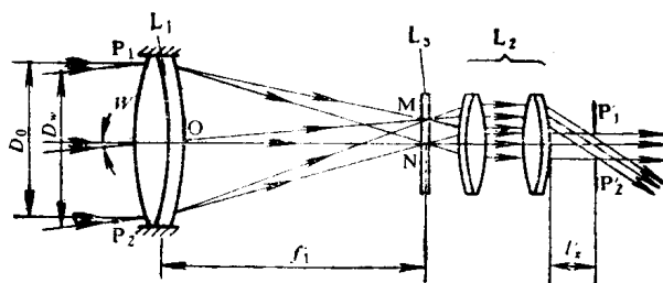
图7-6 望远镜系统的孔径光栏
