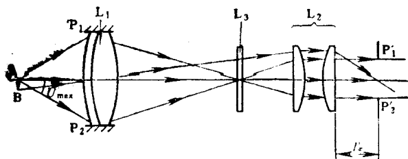
图7-7 简单显微镜的孔径光栏
