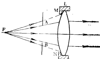
图7-1 孔径光栏在透镜之前
