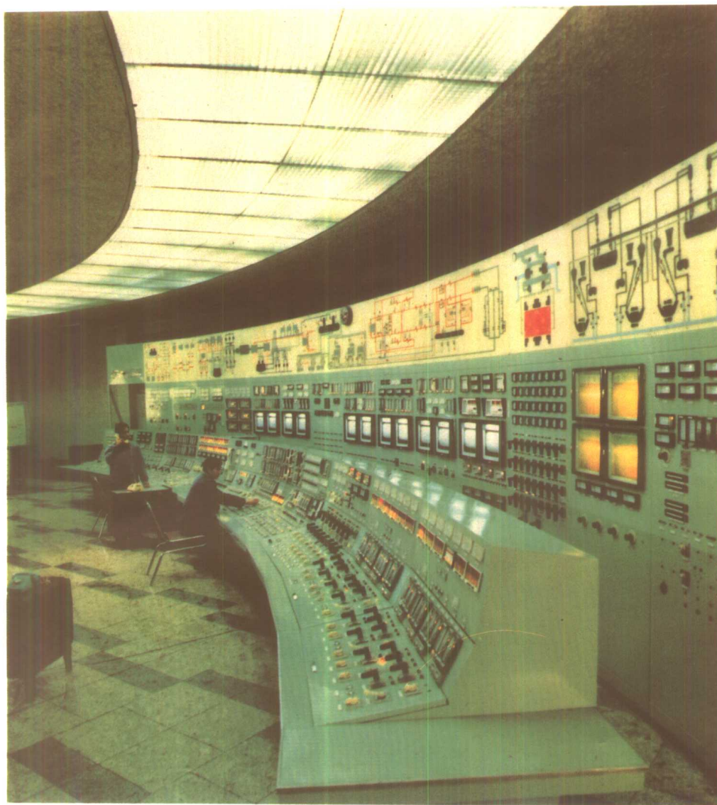
谏壁电站成套仪表
