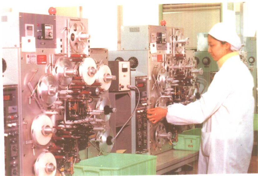
全自动电容器卷绕机
