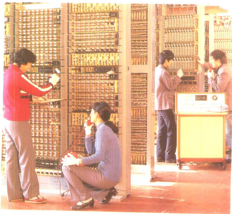
纵横制自动电话交换设备
