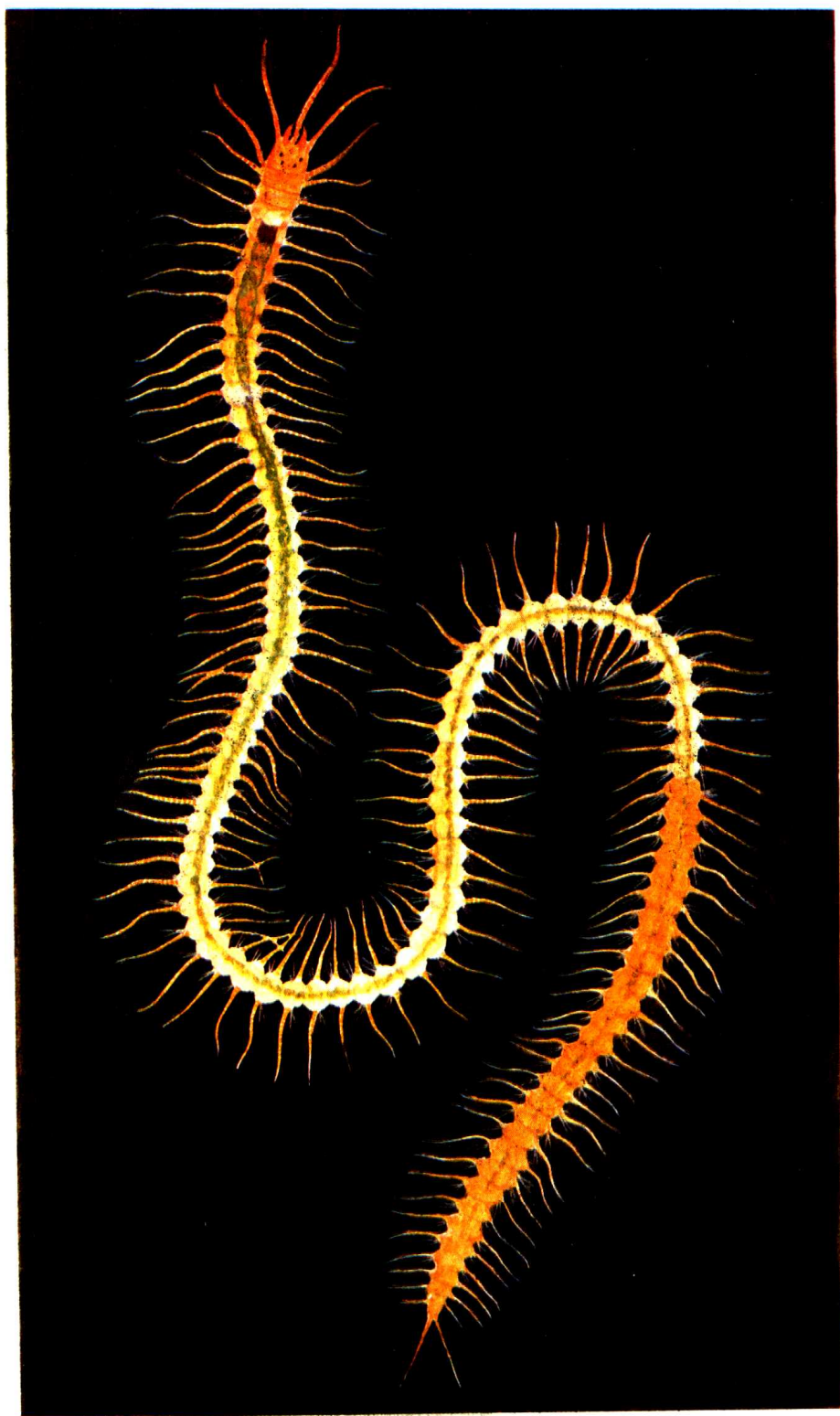
扁模裂虫 Typosyllis fasciata (Malmgren)
