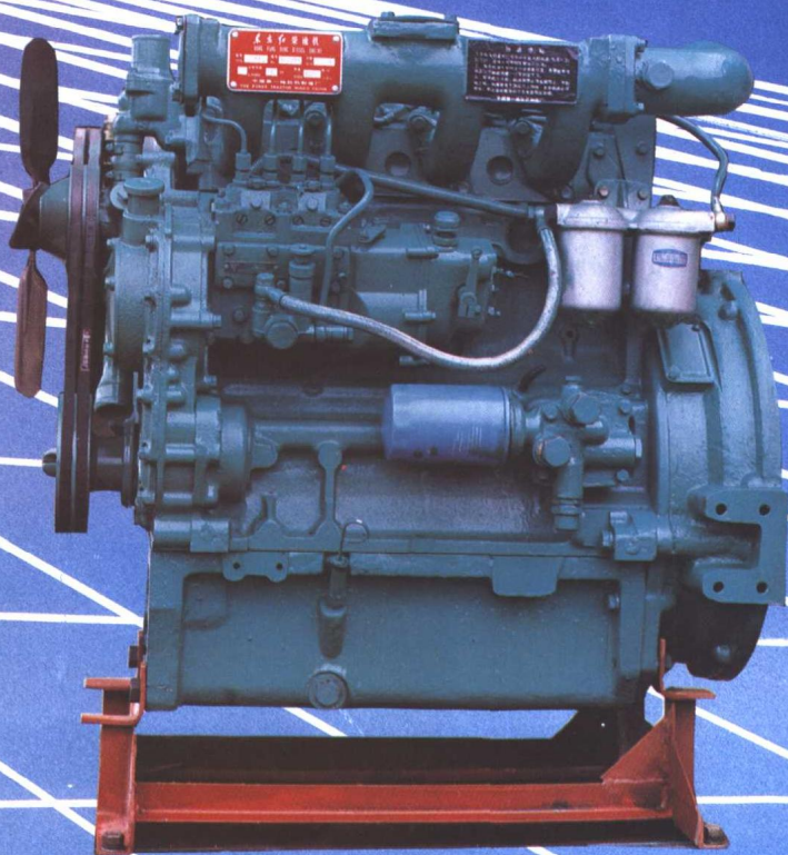
东方红-LR100 柴油机，获省、市、部科技进步一等、二等奖
