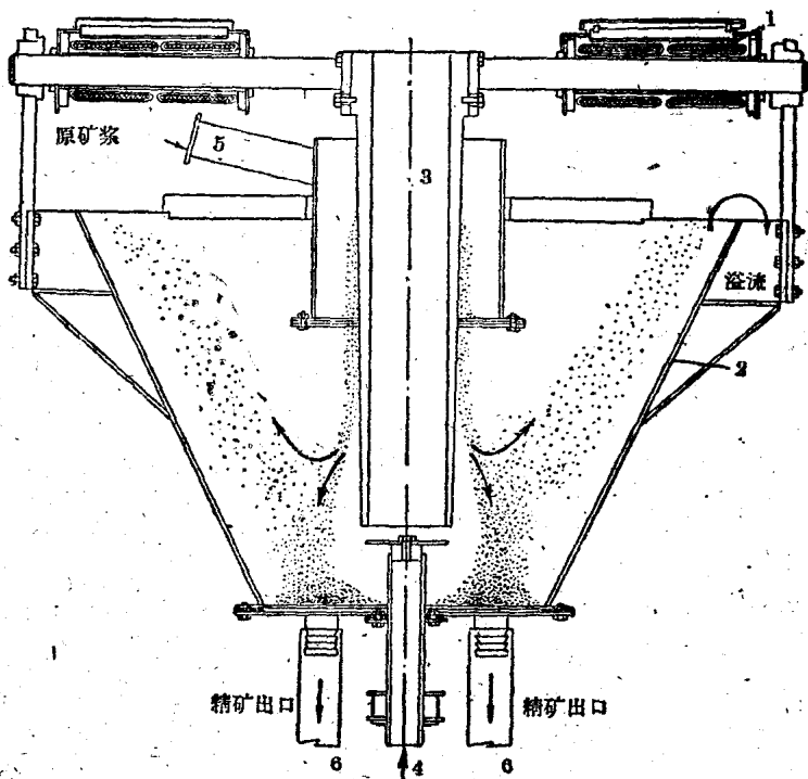
圖 2 磁力脫水槽
