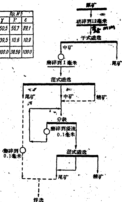
图 4 基姆坎矿床磁铁矿石英岩选别流程
