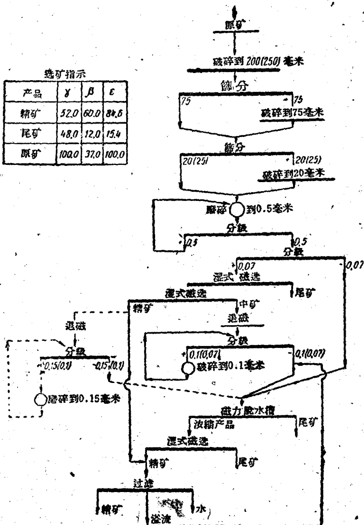
图 1 [斯凯列瓦特磁铁矿] 矿区 (ЮФОР) 磁铁石英岩的合理选矿流程
