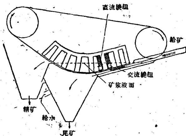
图 5 有脉动磁场 (恒定磁场和交变磁场) 的带式磁选机示意图
