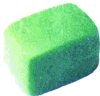
长方体
