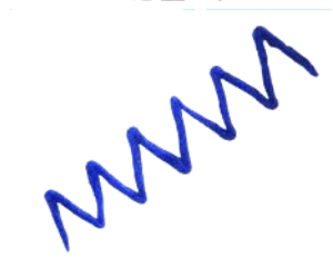
螺旋线
