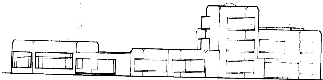
东立面图
