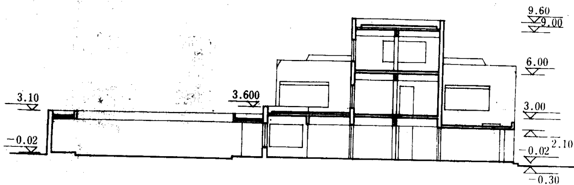
剖面图
