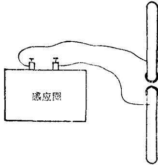
图2 赫兹振子(∨)
