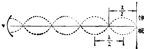
图 6 驻波
