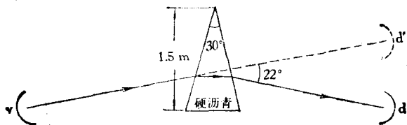
图 5 折射
