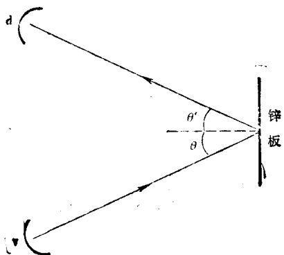
图4 反射
