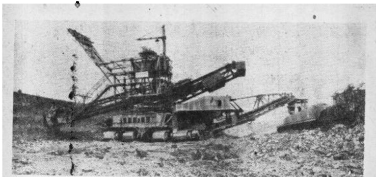
能同時進行掘土和裝土的“克——1000”型巨大掘土機在露天煤礦上工作，它每年能掘土二百五十萬公方。
