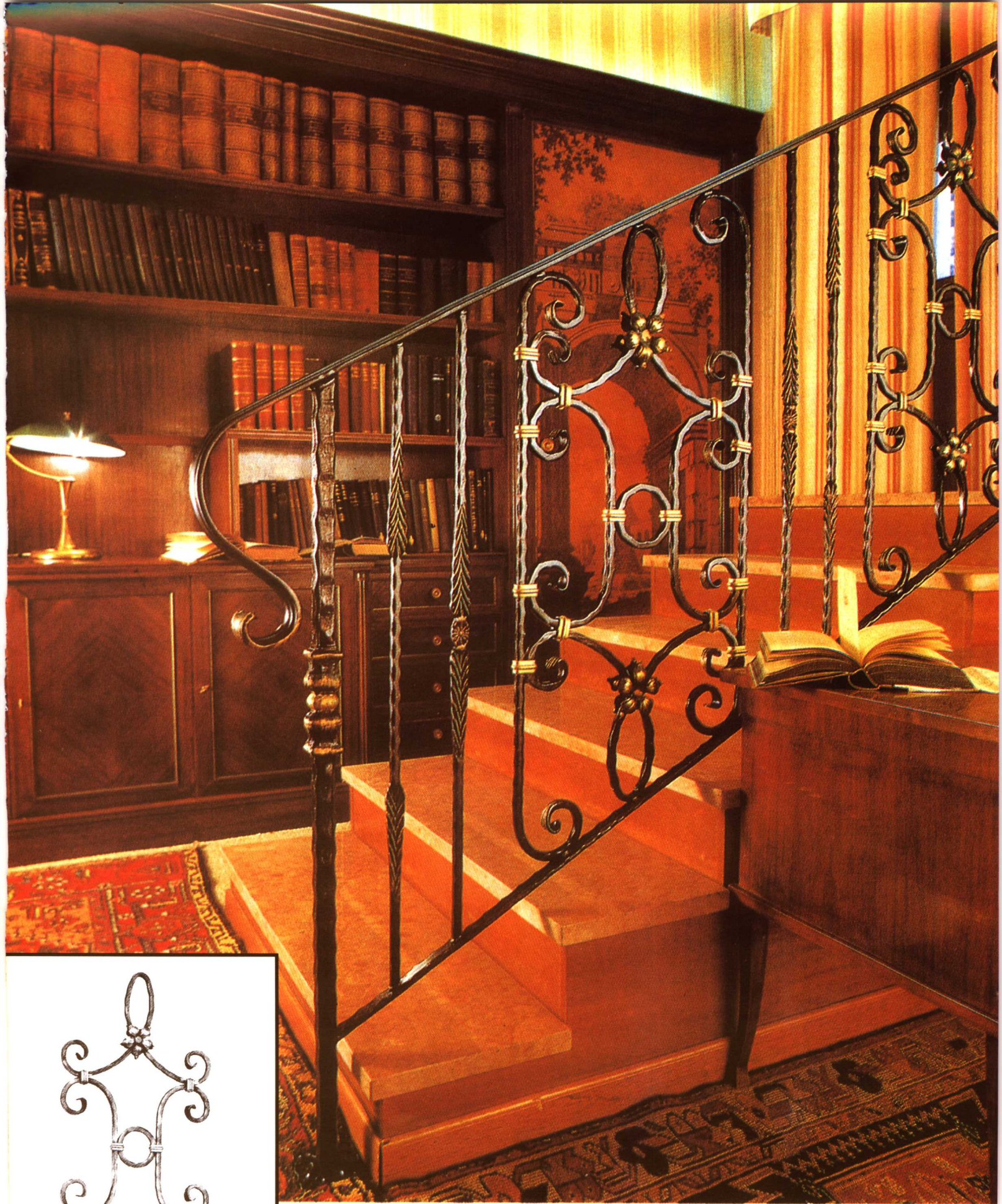
铁艺锻件基本单元: 385 × 900mm
