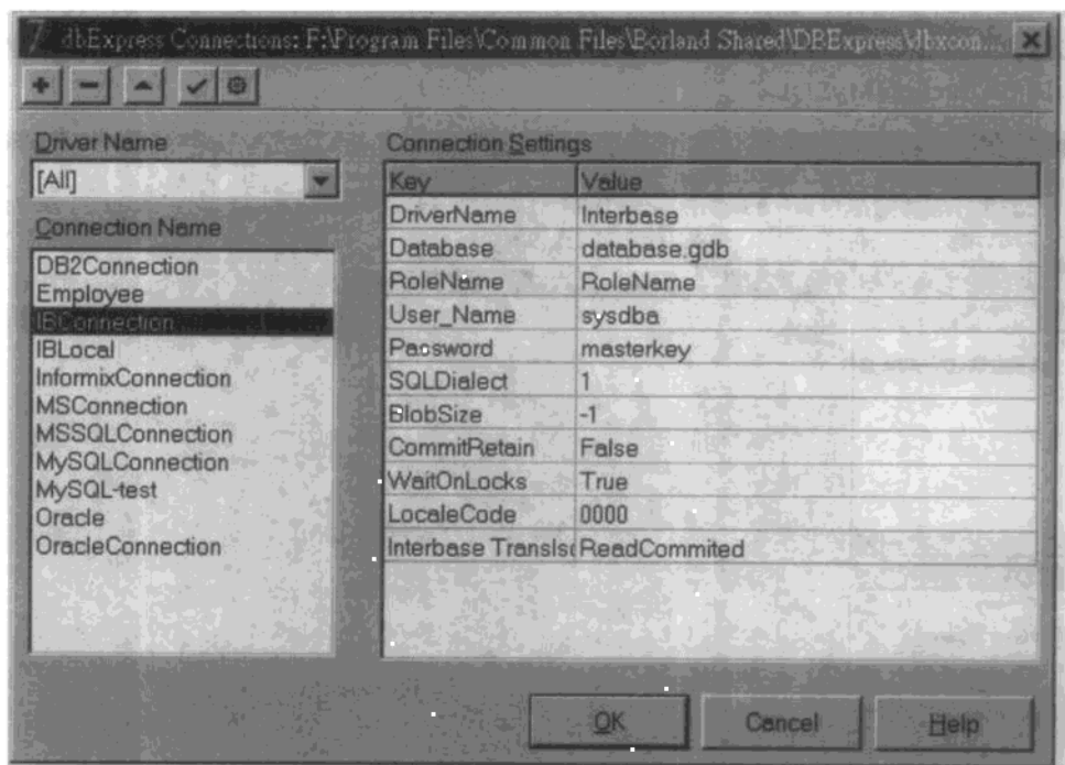
图1-3 TSQLConnection组件的组件编辑器
