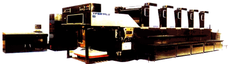
图4 北人 YP5BIMLU 型对开 5 色胶印机
