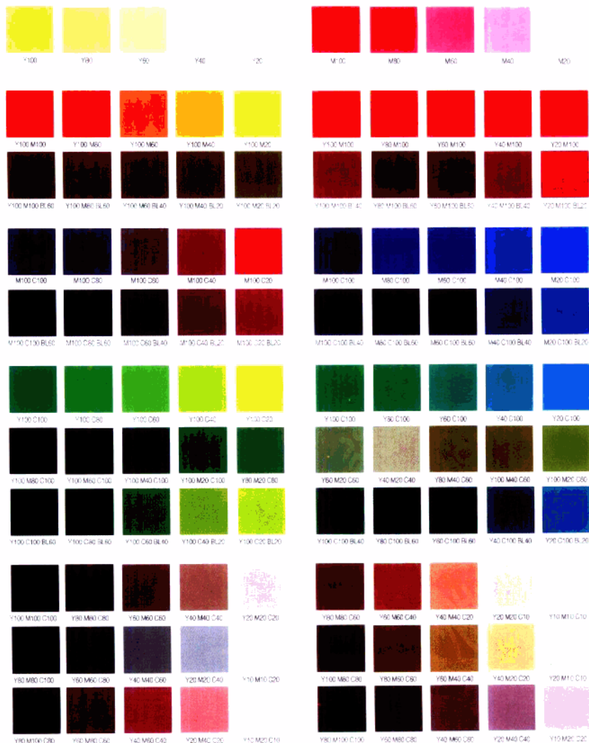
图 7 色谱
