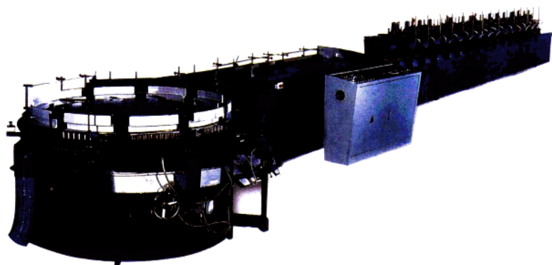
图 13 紫光 BBYL410 圆盘包本联动机
