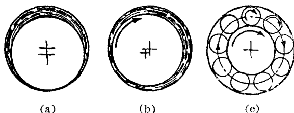
(a) (b) (c) 圖 1-1 滑行與滾行二種軸承之不同作業
