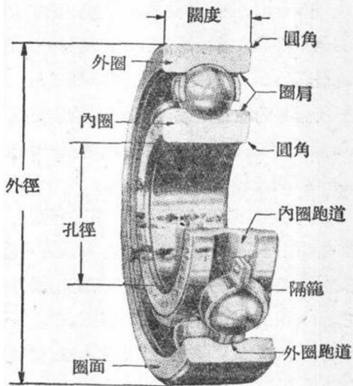
圖 1-2 滾行軸承的基本結構剖面
