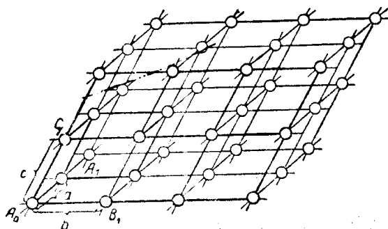
圖1. 晶體的空間格子。
