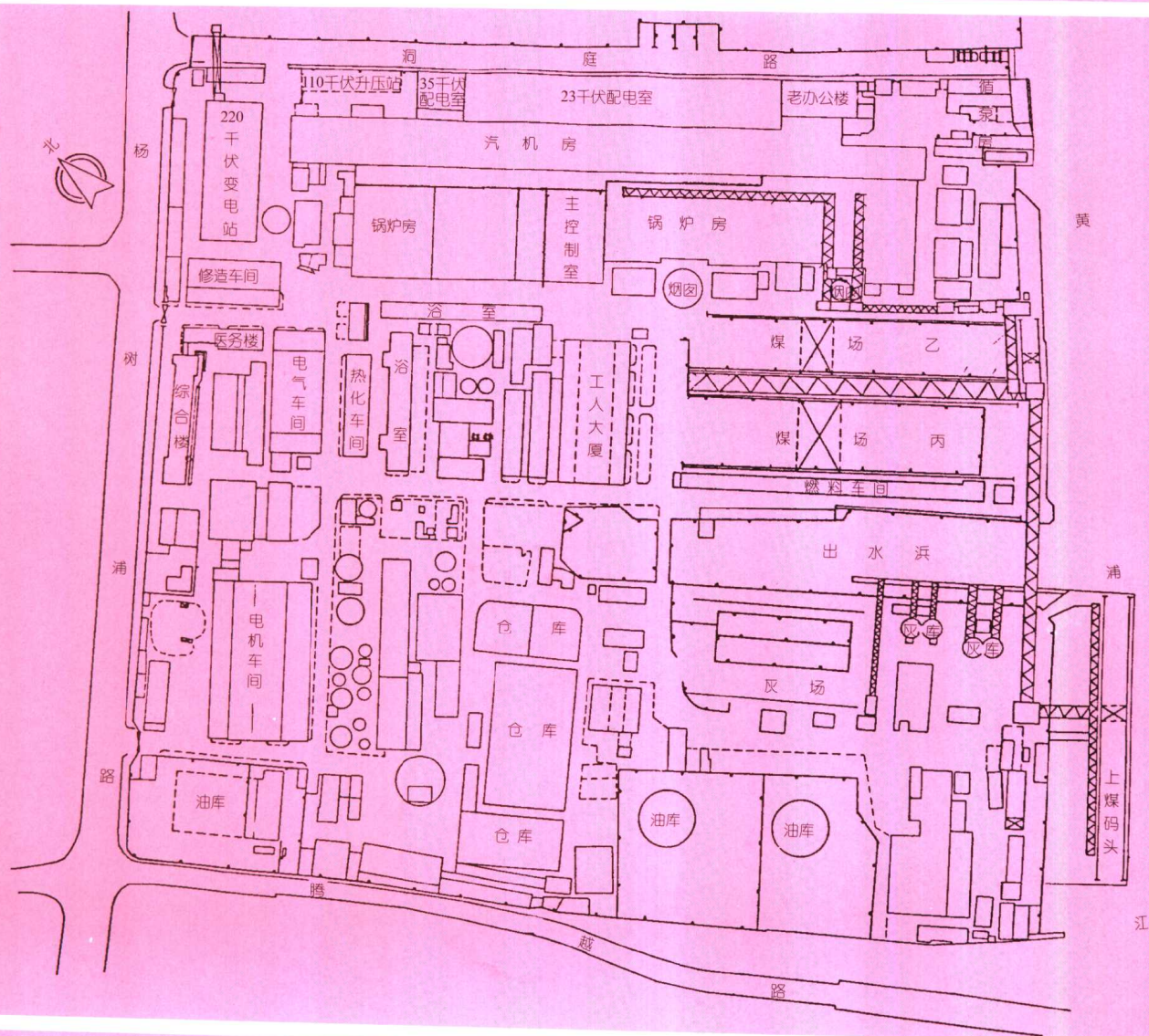
1990年上海杨树浦发电厂厂区图
