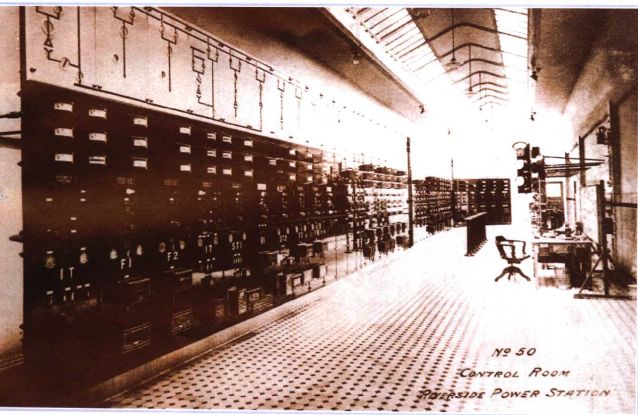
民国13年(1924年)建成的江边电站控制室
