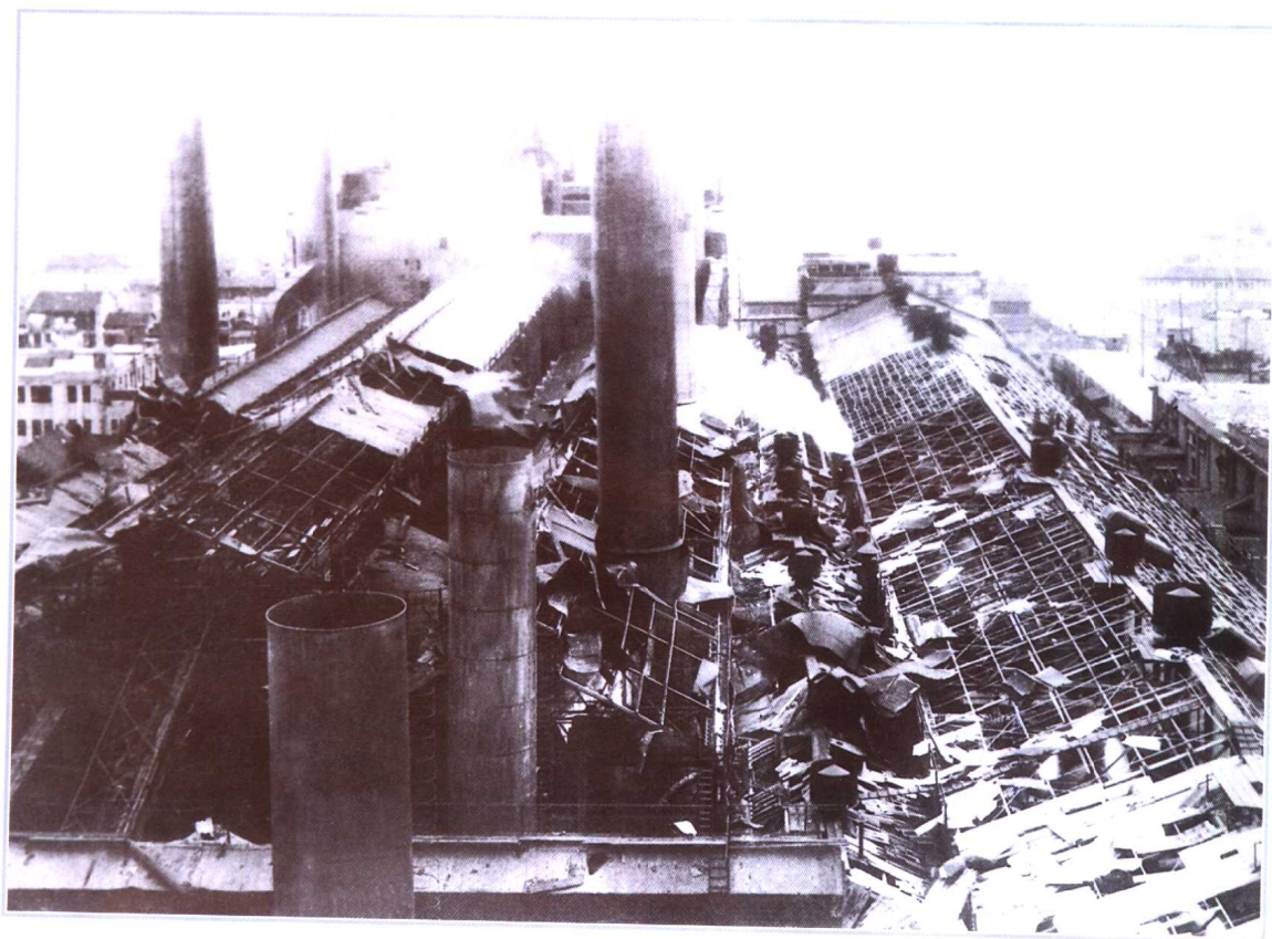
1950年“二·六”轰炸后，二、三号锅炉房及汽机房屋面受损情况
