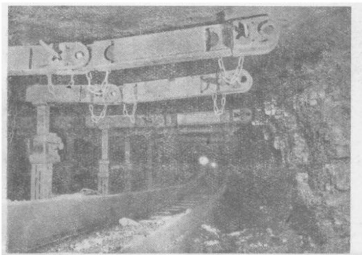
這是蘇聯“羅斯托夫煤炭”聯合廠第二十號煤井中現代化的煤洞。 這裏採用一種金屬移動支架，它能完全保證地下工作的安全。
