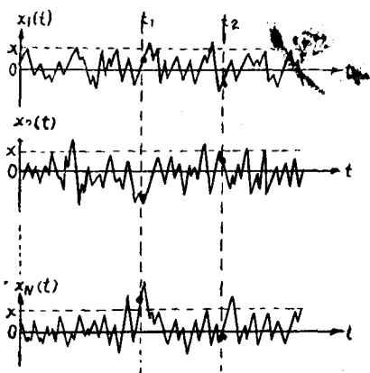
图2.1 样本函数
