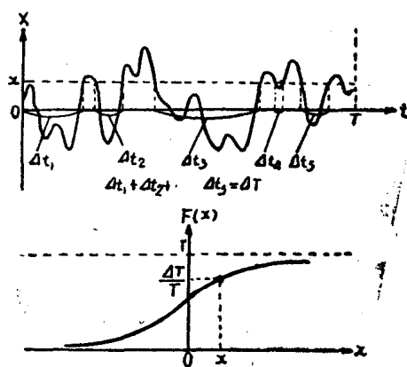
图 2.5 各态历过程的概率分布函数
